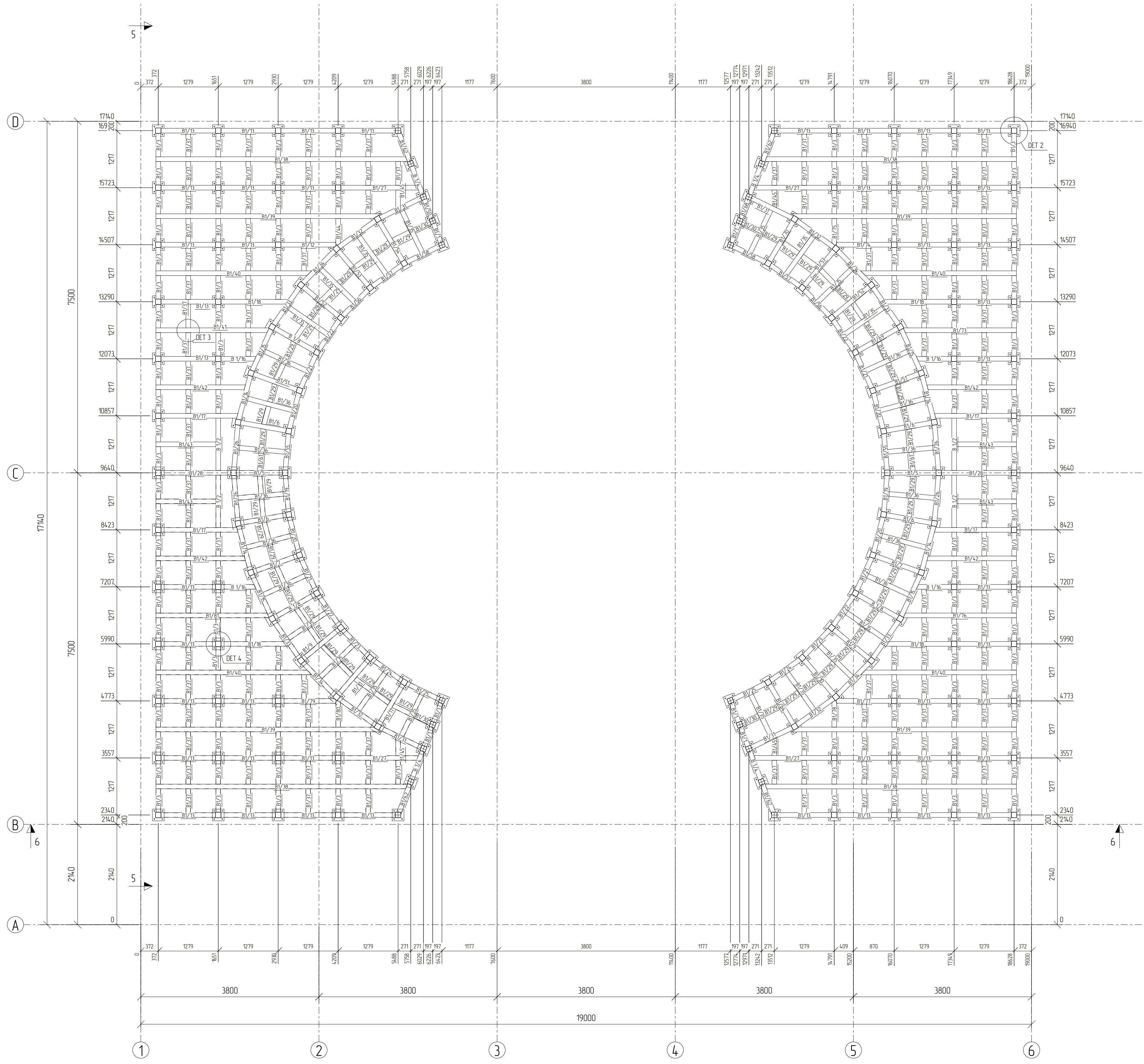
KIRIS YERLEŞİM PLANI
