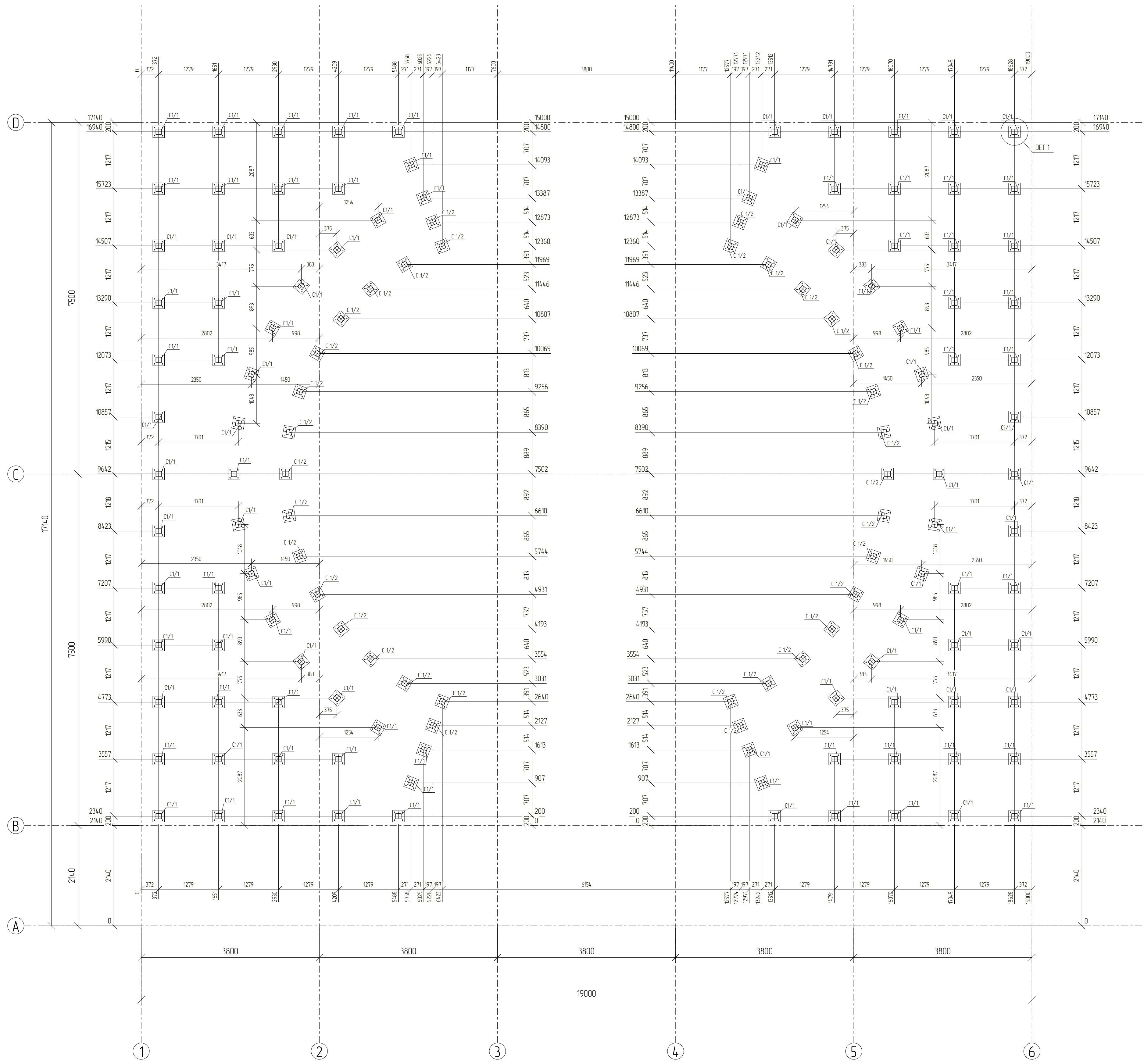
KOLON YERLEŞİM PLANI
