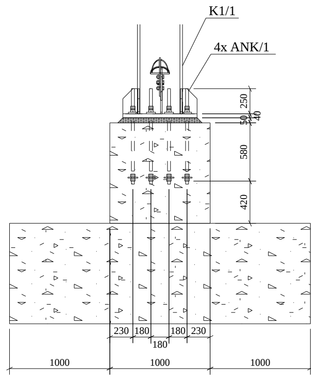
1 KESIT / SECTION Olcek/Scale: 1:50
