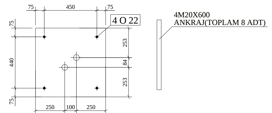
HEA300 SABLON PLAKA DETAYI(2ADT)
