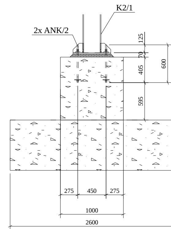
4 KESIT / SECTION Olcek/Scale: 1:50
