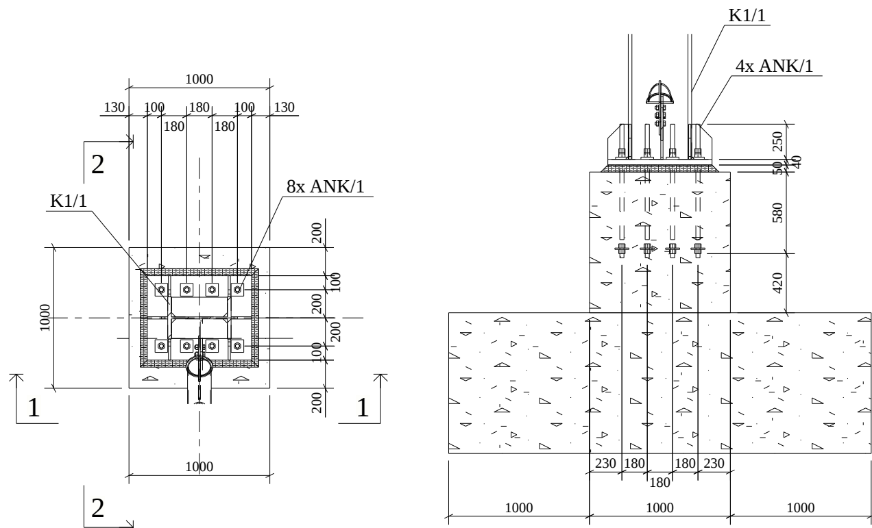
1 KESIT / SECTION Olcek/Scale: 1:50
