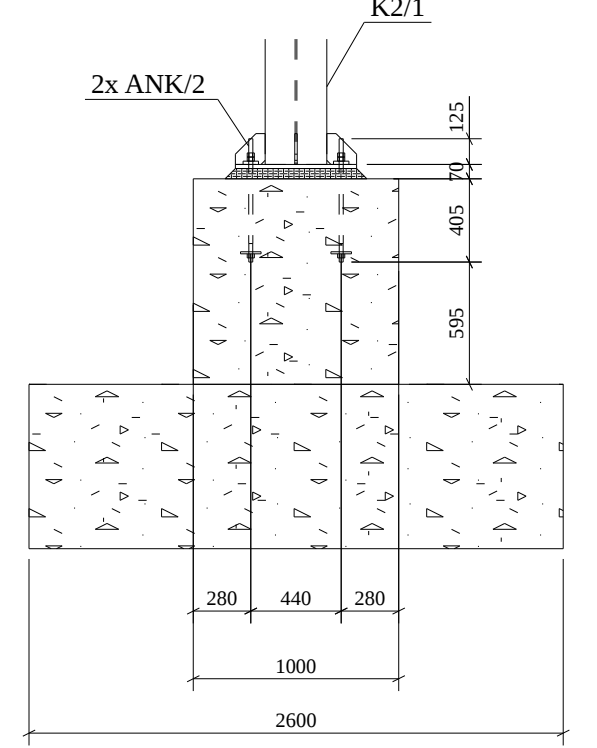
3 KESIT / SECTION Olcek/Scale: 1:50
