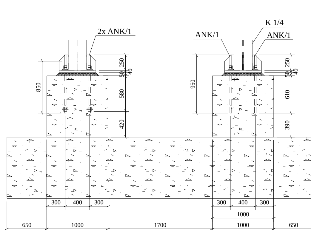
2 KESİT / SECTION Olçek/Scale: 1:50
