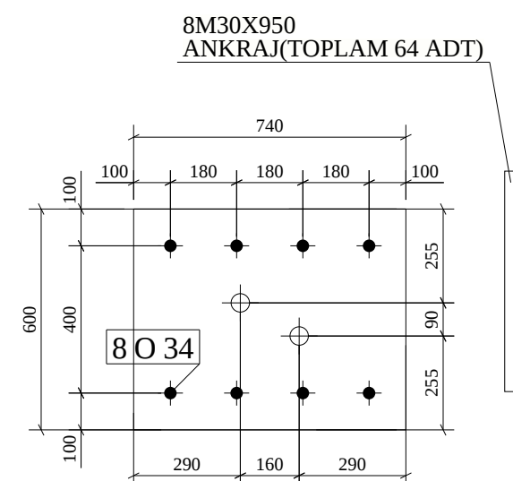
HEB450 KOLON PLAKA DETAYI(8 ADT)
